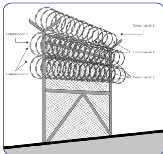
Montaje de concertinas sobre malla metalica
