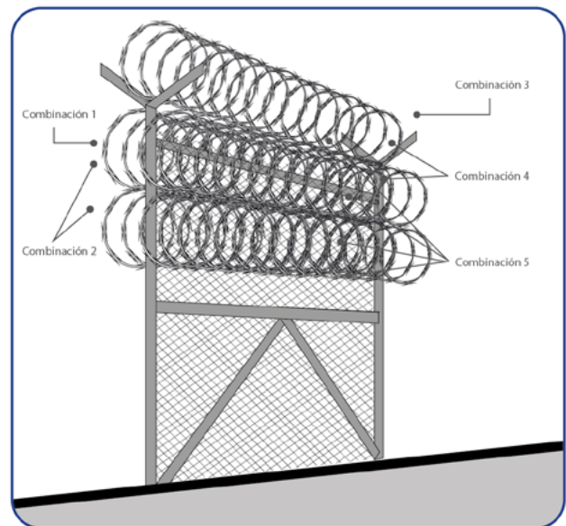
Montaje de concertinas sobre malla metálica
