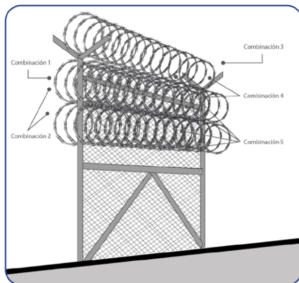
Montaje de concertinas sobre malla metálica
